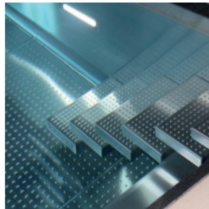
FREITRAGENDE TREPPE
